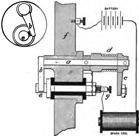
FIG. 37.—Hammer Break.
